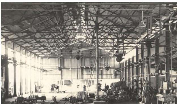
Dit was een van de loodsen van de raffinaderij.
